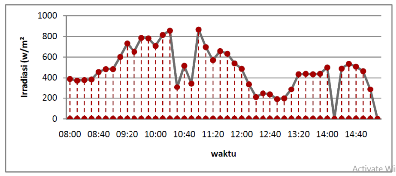
Gambar 3. Grafik Hasil Irradiasi Matahari dari Pyranometer
