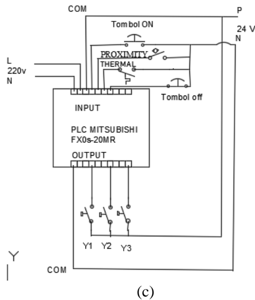
Gambar 2. Wiring diagram rangkaian elektronik mesin injeksi cetak plastik tipe vertikal (a) pengkabelan catu daya, (b) pengkabelan PLC, dan (c) pengkabelan I/O.
