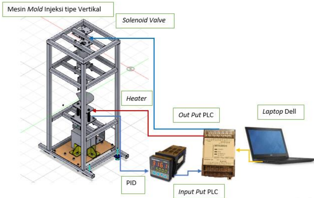
Gambar 3. Rancangan instalasi perangkat pada mesin injeksi cetak plastik tipe vertikal.
