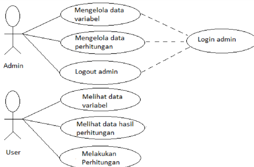
Gambar 3. Use Case Diagram Sistem Online Penentuan Tingkat Kerawanan Longsorlahan
