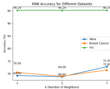
Figure 9. Akurasi KNN terhadap K yang belum dioptimasi
