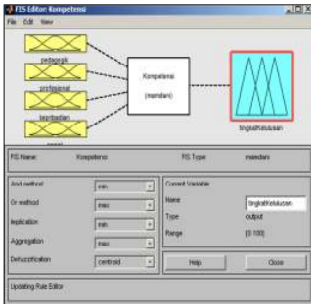
Gambar 9. Sistem inferensi fuzzy Mamdani dengan 4 variabel input dan 1 variabel output
