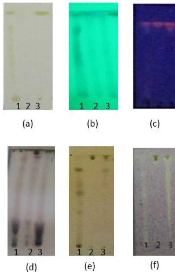
Gambar 2. Kromatogram dengan fase gerak asam format : etil asetat : air = 8 : 1 : 1. KLT fase diam silika gel GF 254 prasalut, (1) ekstrak bunga, (2) ekstrak daun, (3) ekstrak rimpang. (a) visual, (b) di bawah lampu UV \lambda 254 nm, (c) di bawah lampu uv \lambda 366 nm, (d) penampak bercak H 2 SO 4 10%, (e) penampak bercak FeCl 3 , (f) DPPH 0,2% dalam metanol.
