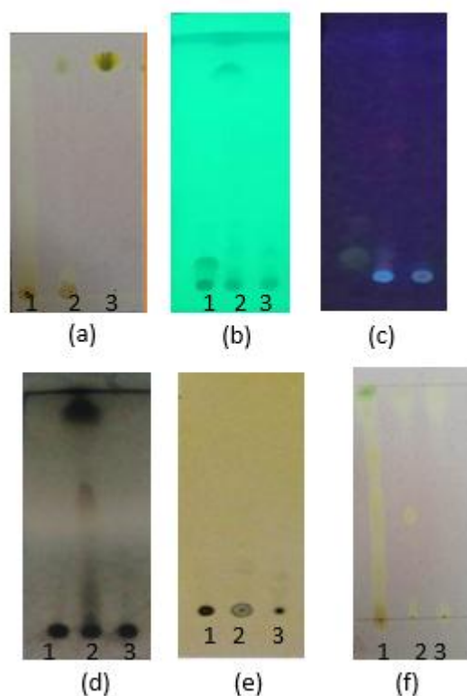
Gambar 1. Kromatogram ekstrak dengan fase gerak n-heksana : etil asetat = 8 : 2. KLT fase diam silika gel GF 254 prasalut, (1) ekstrak bunga, (2) ekstrak daun, (3) ekstrak rimpang. (a) visual, (b) di bawah lampu UV \lambda 254 nm, (c) di bawah lampu uv \lambda 366 nm, (d) penampak bercak H 2 SO 4 10%, (e) penampak bercak FeCl 3 , (f) DPPH 0,2% dalam metanol.
