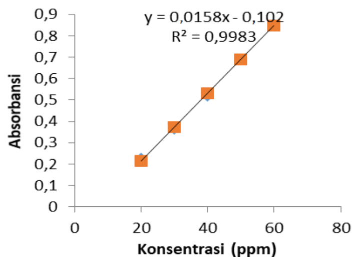
Gambar 3. Kurva kalibrasi DPPH.
