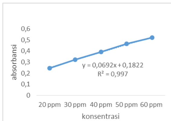
Gambar 4. Kurva kalibrasi asam galat.
