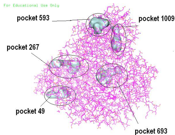
Gambar 1. Visualisasi lima pocket terbaik pada 2QMJ.
