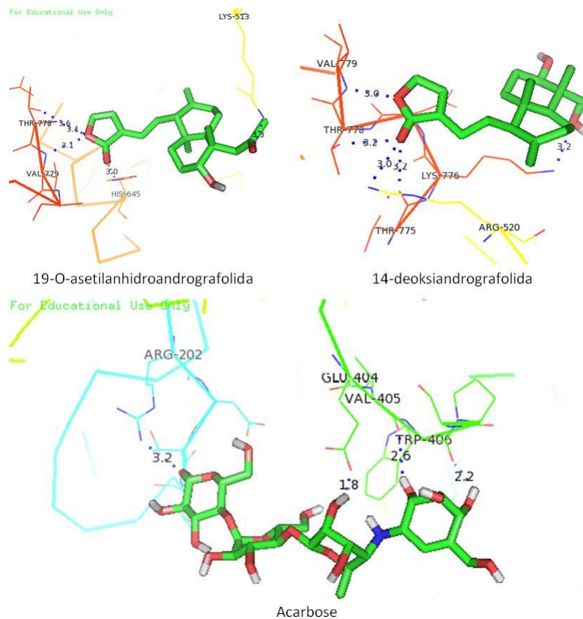
Gambar 2. Kontak residu pada 19-O-asetilanhidroandrografolida, 14-deoksiandrografolida dan acarbose.
