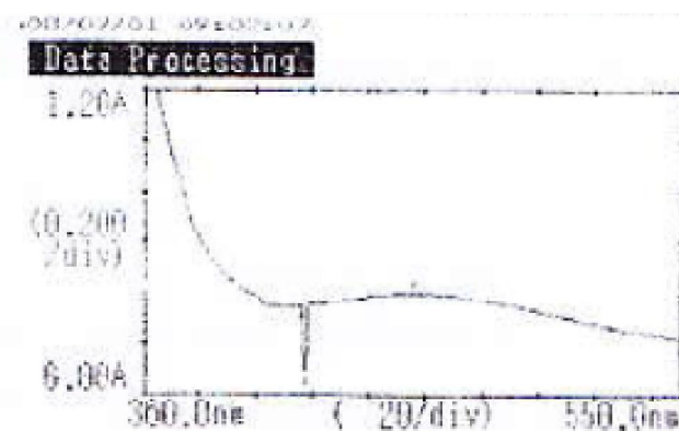
Gambar 1. Scanning kompleks (\text{Fe}(\text{SCN}))^{2+} dengan NaCl
