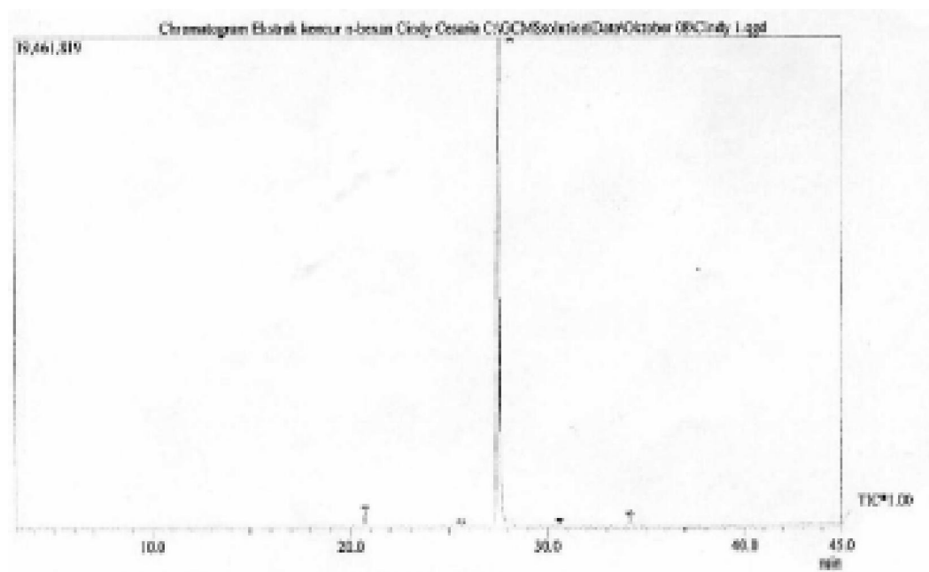
Gambar 1. Hasil kromatogram ekstrak kencur dengan pelarut N-heksan menggunakan Kromatografi Gas.
