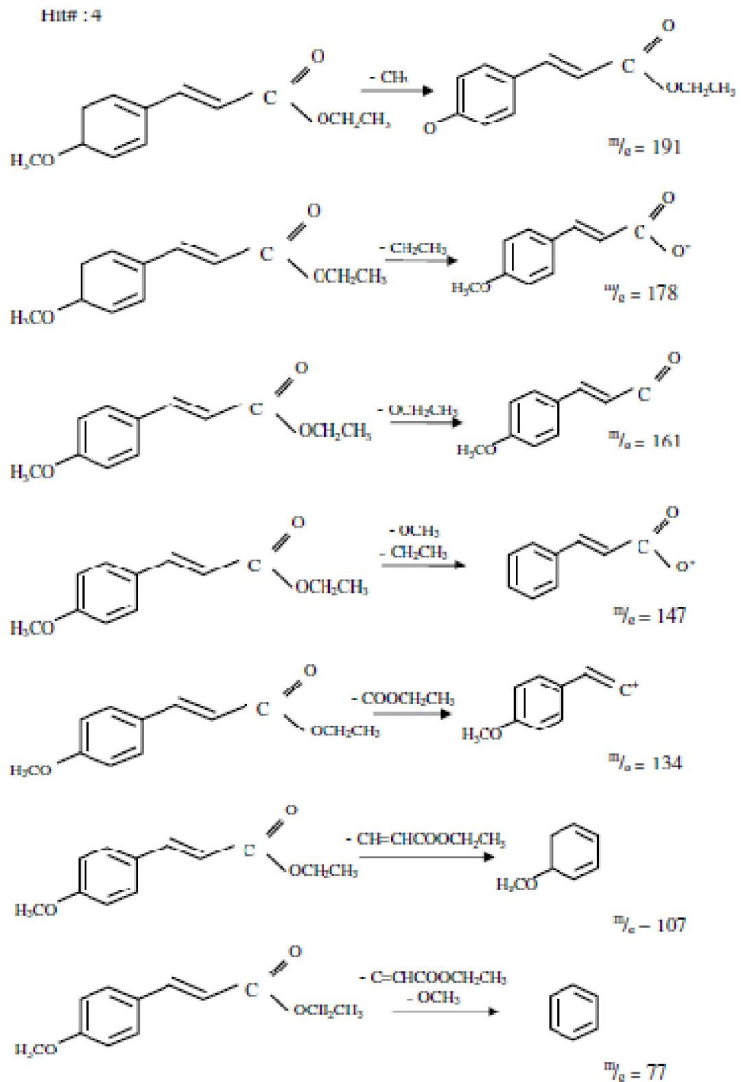
Gambar 3. Perkiraan Pola fragmentasi Spektroskopi Massa yang menunjukkan kemungkinan terdapatnya EPMS pada hit#3.
