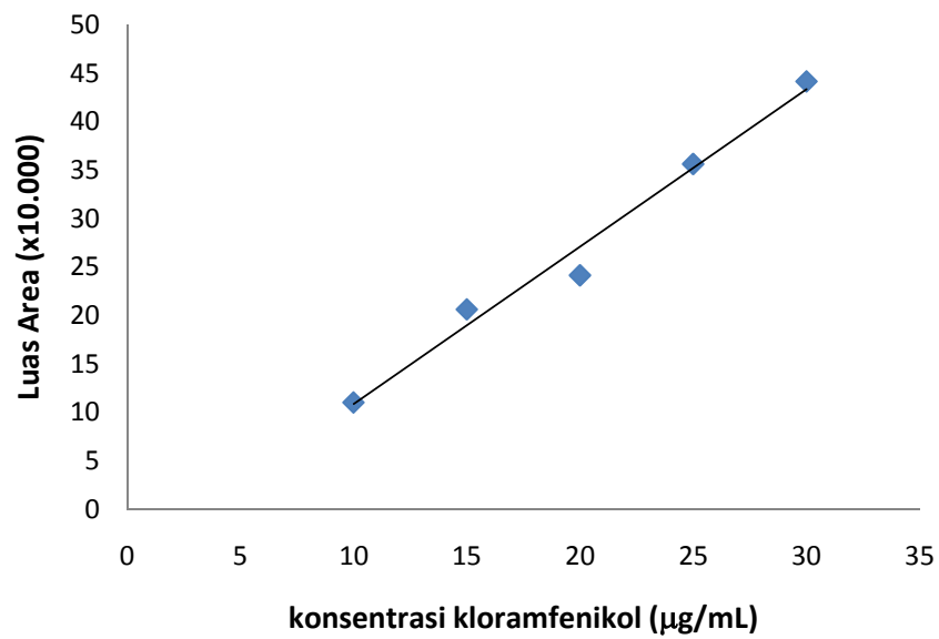
Gambar 2. Kurva hubungan konsentrasi kloramfenikol (µg/mL) dan luas area
