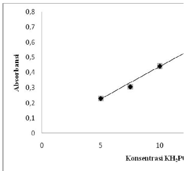
Gambar 2. Kurva baku hubungan konsentrasi KH 2 PO 4 dengan absorbansi
