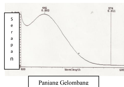
Gambar 1. Scanning Panjang gelombang Larutan Dikromat Asam
