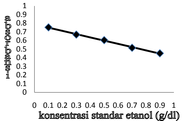
Gambar 2. Kurva hasil Pembuktian Hukum Lambert Beer
