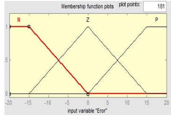
Gambar 6. Fungsi keanggotaan variabel error
