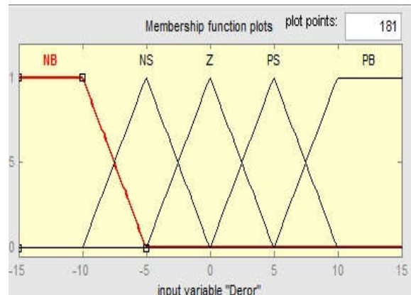
Gambar 7. Fungsi Keanggotaan Variabel Derror
