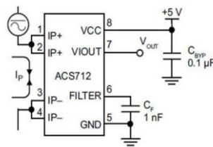
Gambar 2 Rangkaian Sensor Arus
