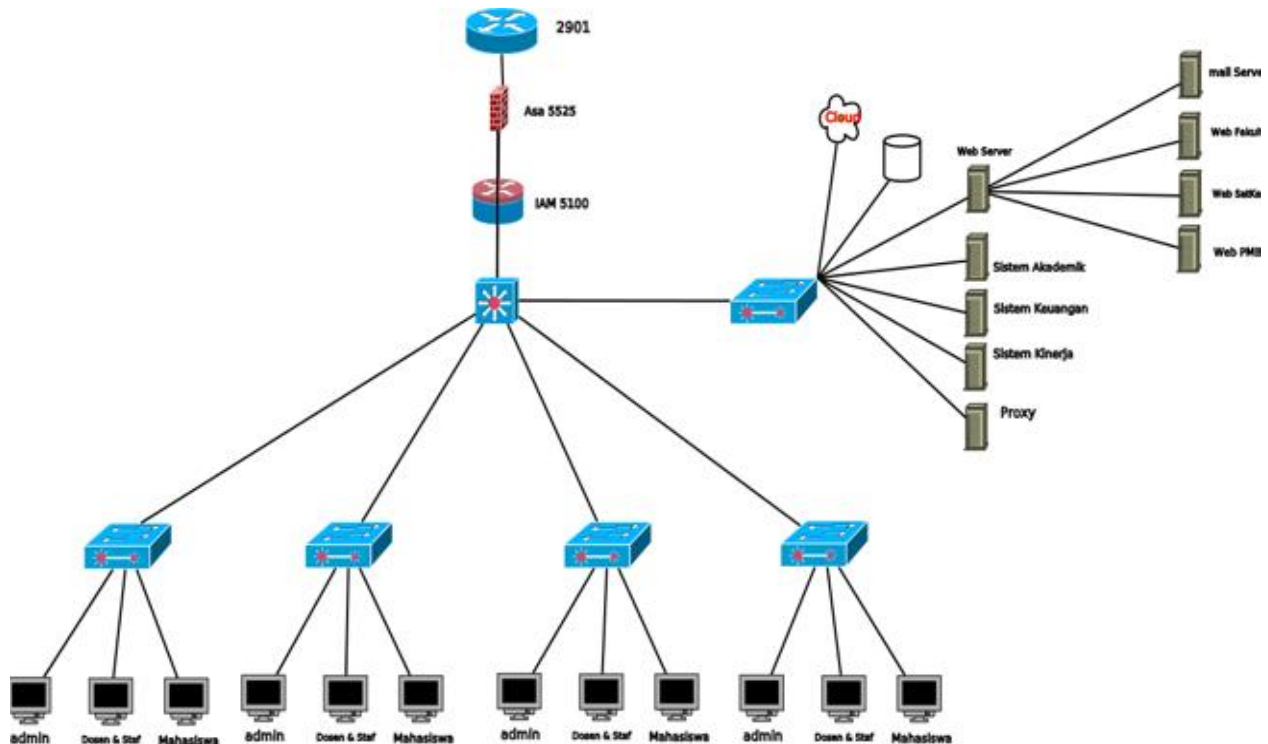
Gambar. 2. Topologi yang digunakan
