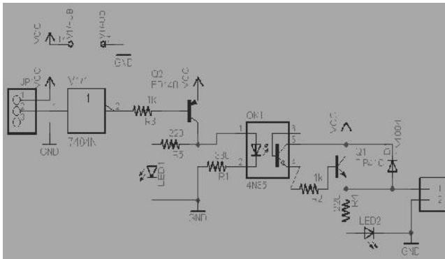
Gambar 5. Skema keluaran magnetic encoder
