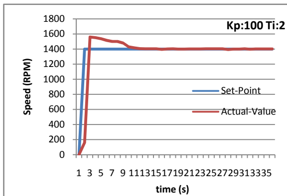
Gambar 11. Kurva Respon Sistem Kendali Proporsional-Integral (PI) pada Setpoint 1400 RPM dengan nilai Kp=100 dan Ti=2
